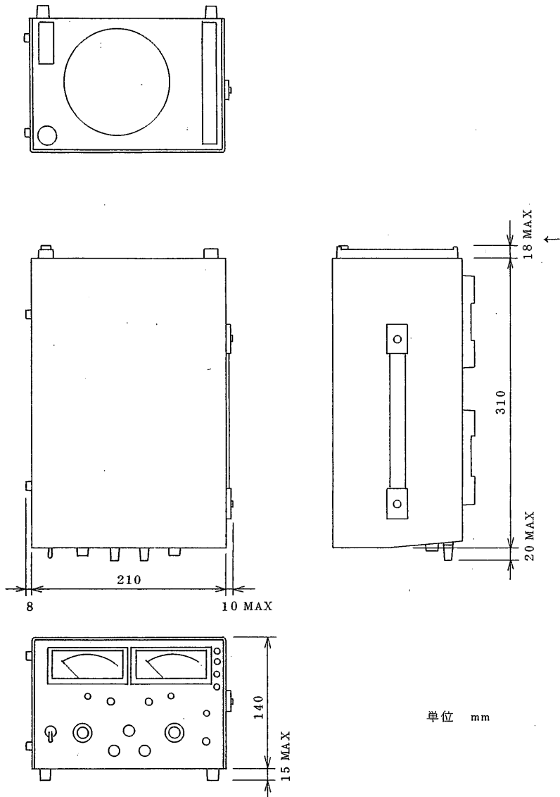
[ 图 1-1 ] 外形图
